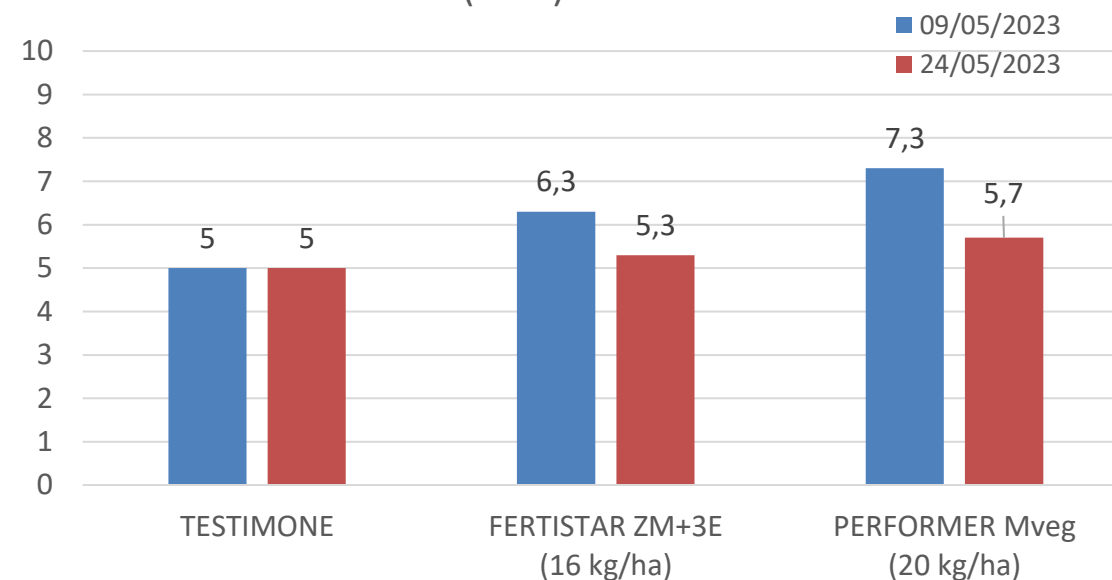
VIGORE (1-10) – TESTIMONE = 5
