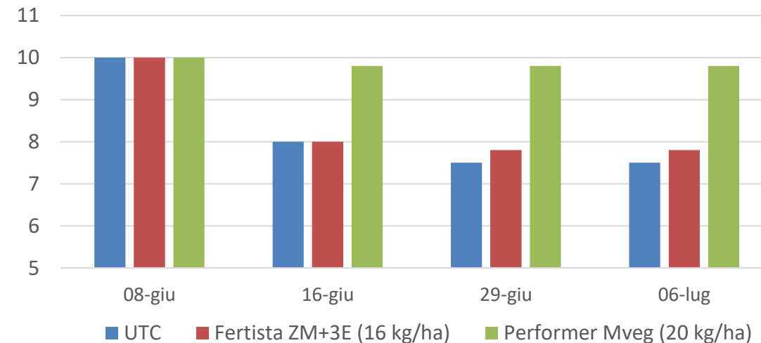
VIGORE (0-10)
